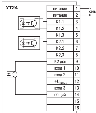
Рис. Б.3. Подключение прибора модификации УТ24–Х.К
